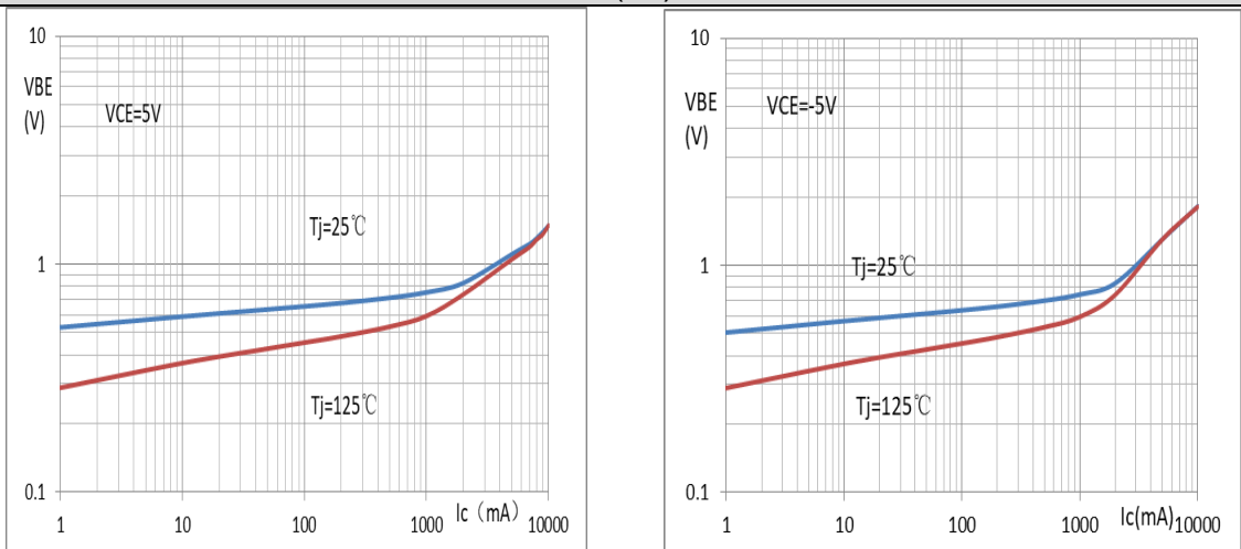
VCE(sat)-Ic
