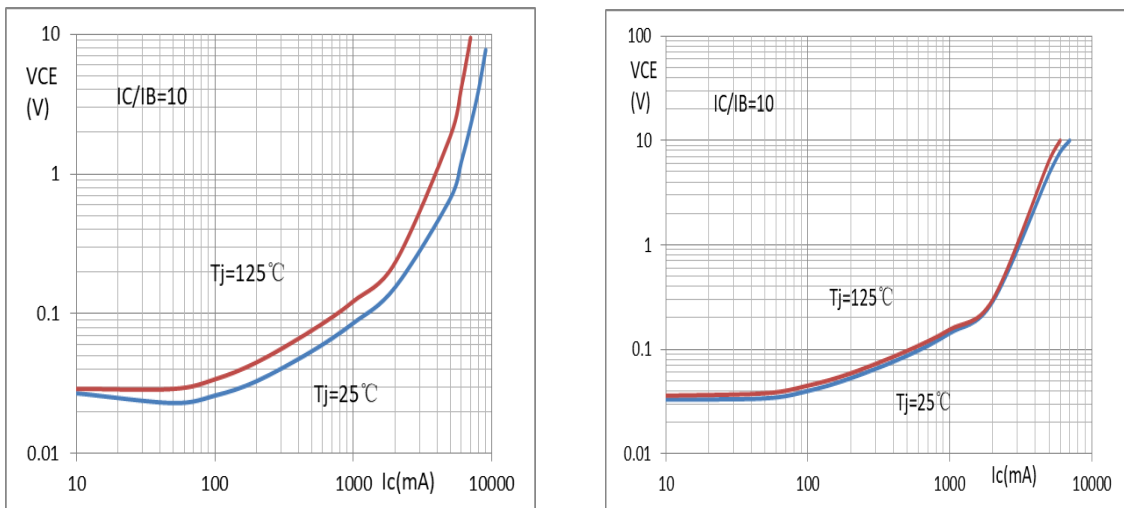
VCE(sat)-Ic
